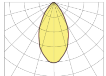
Circulaire 50° (C5)
