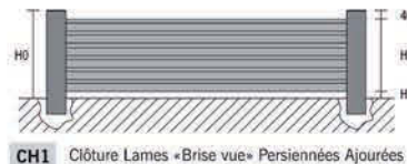
CH1 Clôture Lames «Brise vue» Persiennées Ajourées
