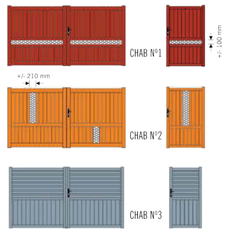
LAMES «Z» OU BRISE-VUE SIMPLE + SOUBASSEMENT LAMES PLEINES
