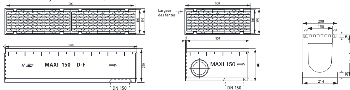
Caniveau avec 2 grilles de couverture, section d'entrée 736 cm 2 /m
