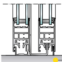
Patin de guidage à point fixe latéral
