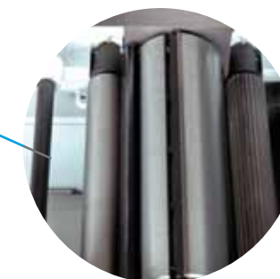
Rouleaux d'entraînement ø 40 mm pour l'avance de la pièce de bois. Arbre de 95 mm à 4 fers Voedingsrollen met ø 40 mm om het stuk hout voort te bewegen. As van 95 mm met 4 messen
