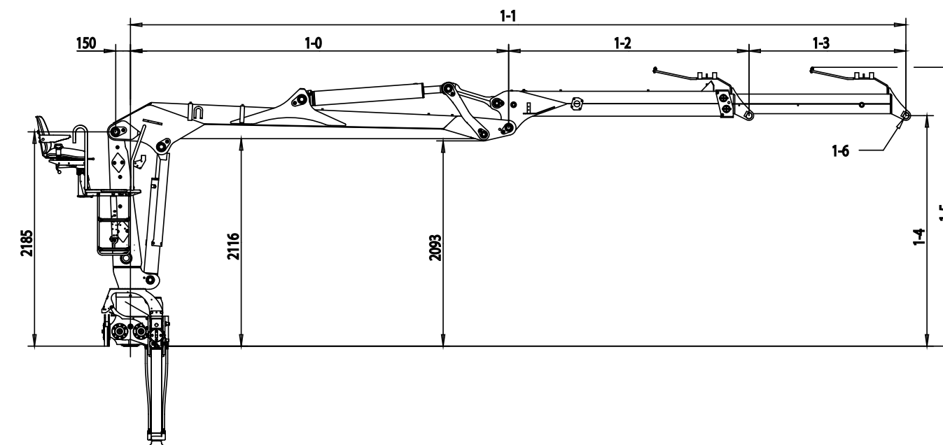
Vue latérale
