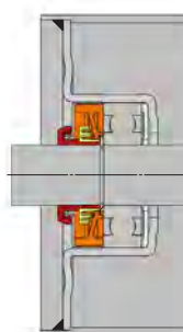
F : Soudure boîtier à aile plate à l'intérieur du tube
