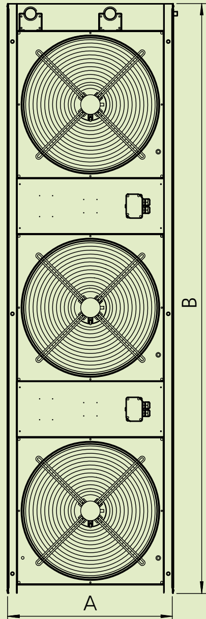
Modèle vertical
