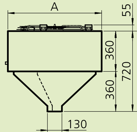
Sortie centrale
