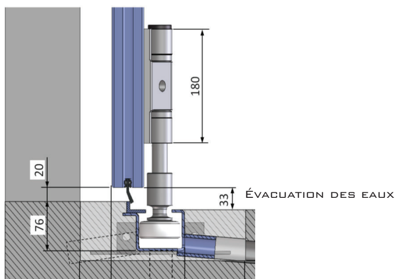
RAIL DE GUIDAGE D'ARRÊT EN- CASTRÉ DANS LE SOL
