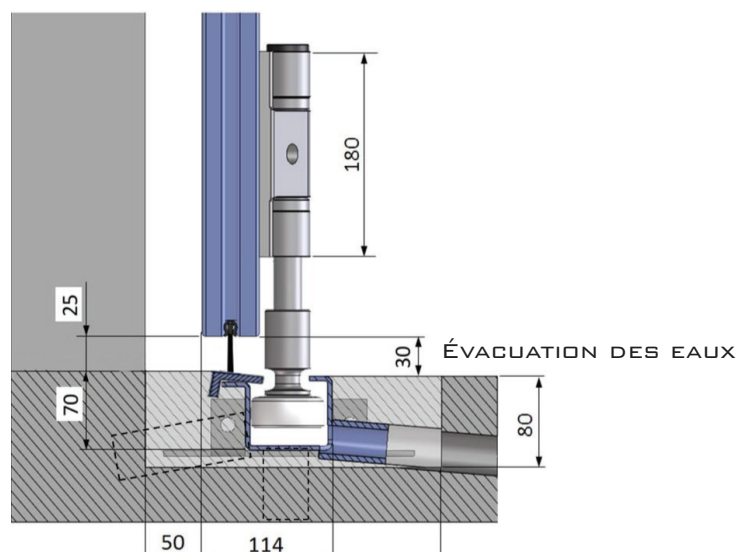
RAIL DE GUIDAGE ENCASTRÉ DANS LE SOL AVEC BUTÉE MINIMUM
