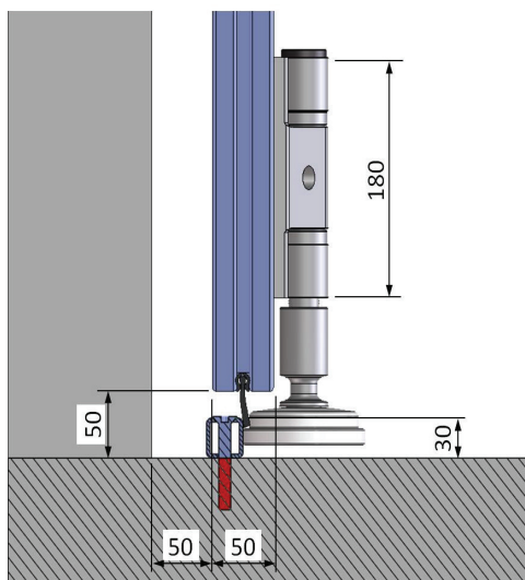
RAIL INFÉRIEUR AVEC SEUIL
