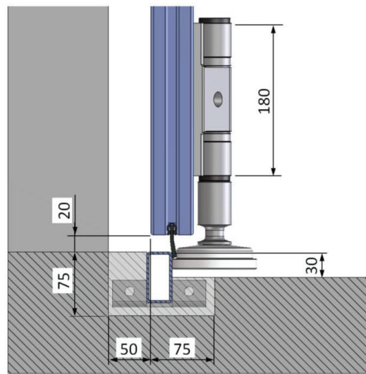
RAIL D'ARRÊT EN- CASTRÉ DANS LE SOL
