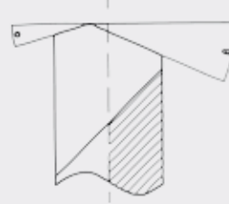
Affûtage 2 pentes
