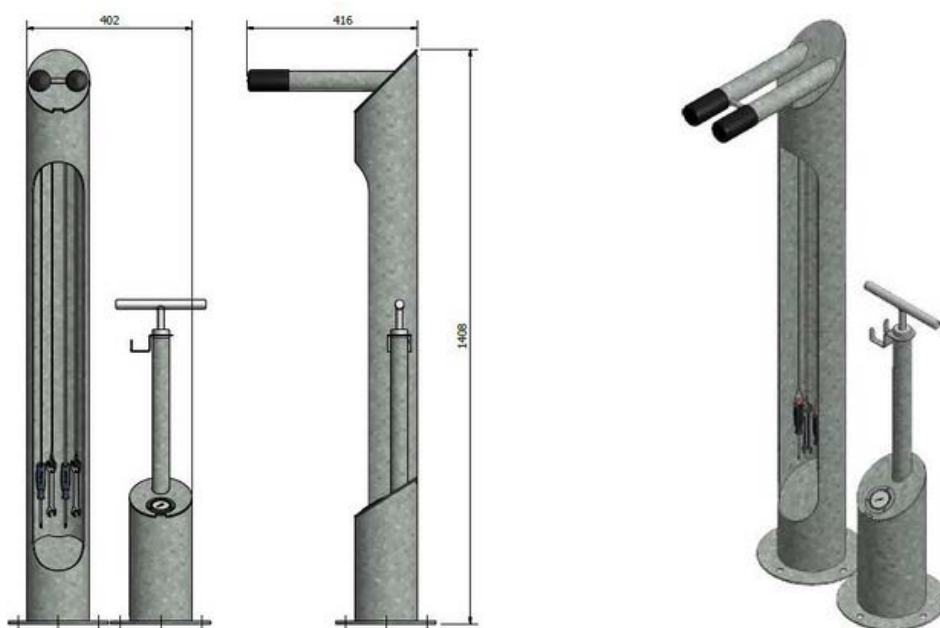
Figure 2. Totem d'outillages et pompe manuelle – Dimensions
