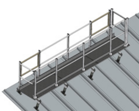
Passerelle sur toiture zinc volige
