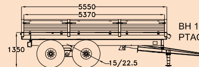
BH 120 PTAC : 16 000 kg
