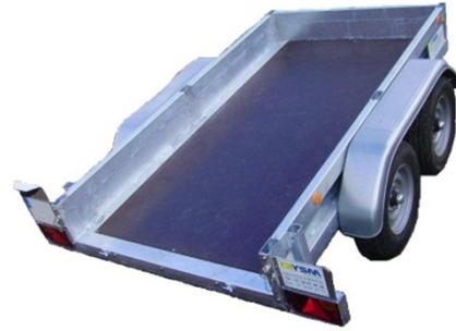
Plateau basculant et RBA - CU 1944 kg
