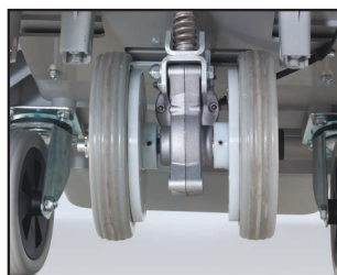
2 roues centrales de traction
