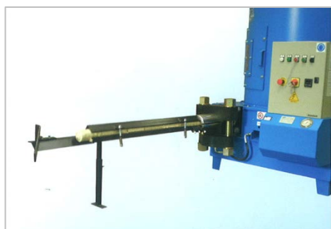
Conduite de refroidissement avec coupe briquette mécanique
