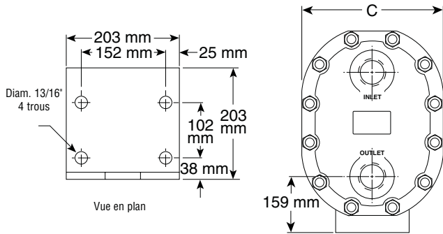
Support de montage au sol pour LS et MS
