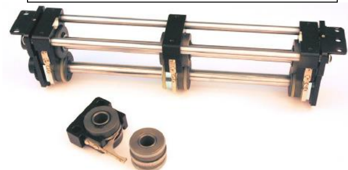
BLOC DE COUPE A COUPEAU CIRCULAIRE
