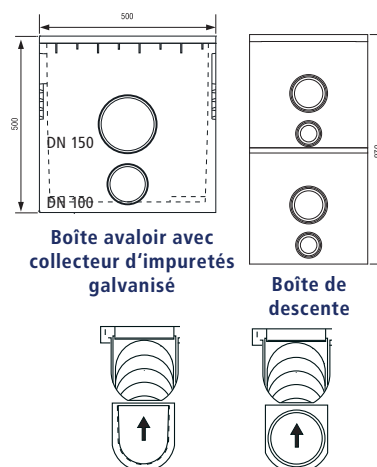
Boîte frontale fermée avec tube DN 100 N° d'art. : 7001110 N° d'art. : 7001120
