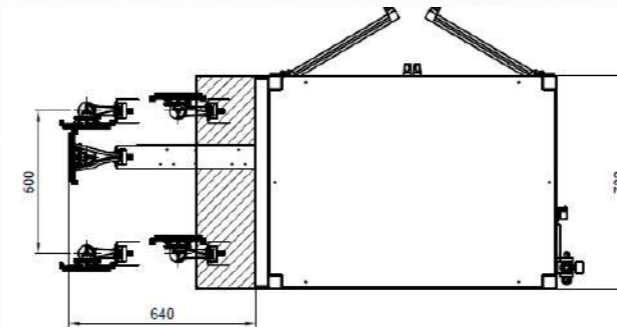
Vue du dessus
