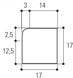
T3 basse
