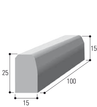
T2 biaisé
