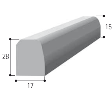
T3 biaise
