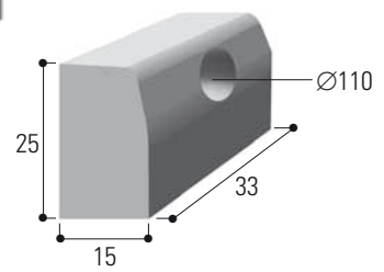
T2 gargouille
