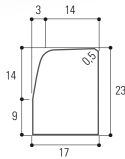
T3 réduite
