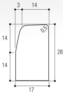
T3
