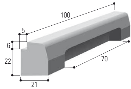
T3 avaloir non traversant
