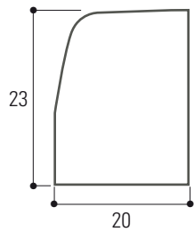
T4 réduite
