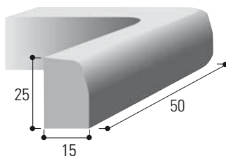
T2 d'angle
