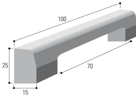
T2 avaloir
