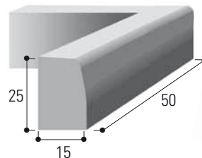
T2 d'angle vif
