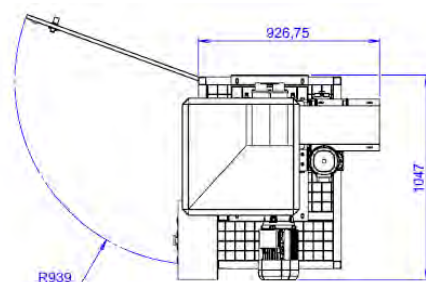
BB230 sortie vis «BLIK» un sac à déchets quelconque s'adapte facilement à la sortie de la vis
