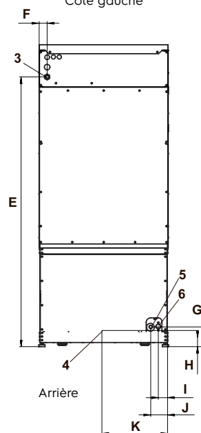
Côté gauche
