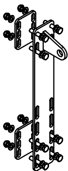
Platine de fixation supérieure Entraxe entre les échelons 250mm < e < 400mm
