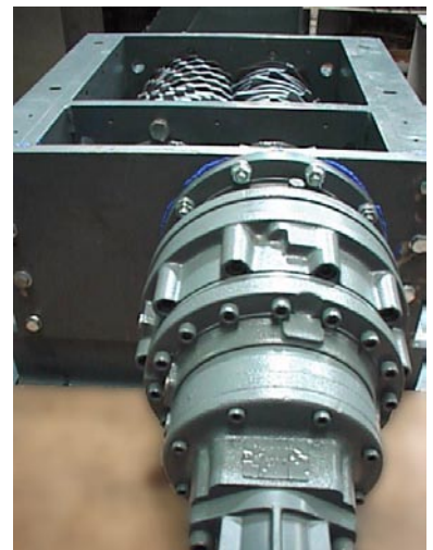
Broyeur B400 spécialement équipé pour installation mobile
