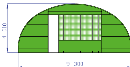
PORTE PARTHENAY
