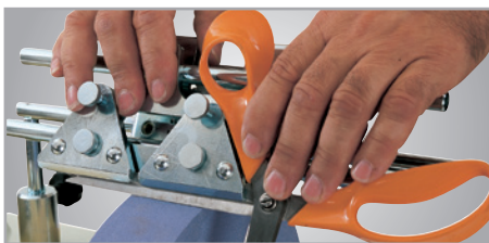
• Dispositif pour ciseaux (code article 591 0058)
