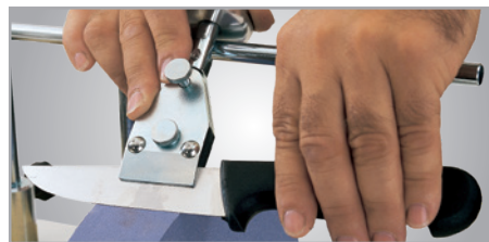
• Dispositif pour couteaux lame courte (code article 576 0056)
