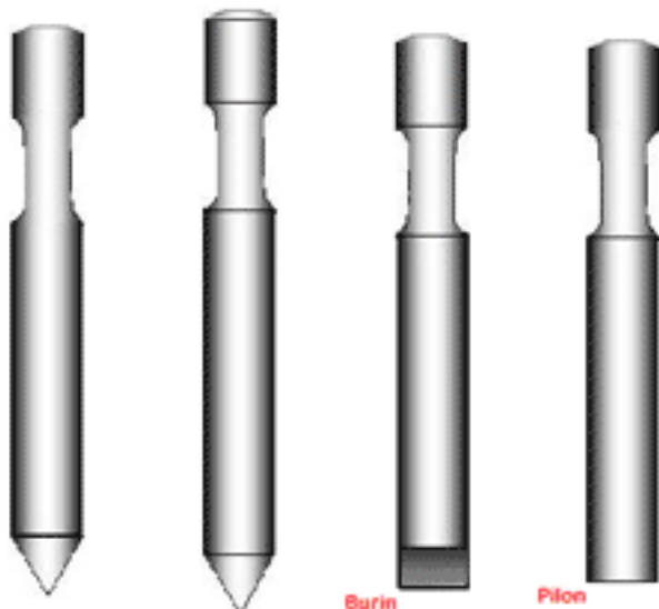
Pic Longueur (mm) 1100 Largeur (mm) 122 Poids (daN) 94 Pic long Longueur (mm) 1300 Largeur (mm) 122 Poids (daN) 109 Barin Longueur (mm) 1100 Largeur (mm) 122 Poids (daN) 94 Pilon Longueur (mm) 1100 Largeur (mm) 122 Poids (daN) 98
