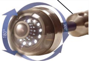
Caméra rotative : Pan 360° x Tilt 180°
