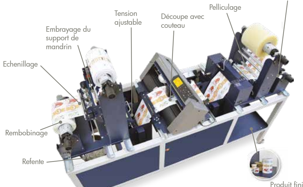
Embrayage du support de mandrin
