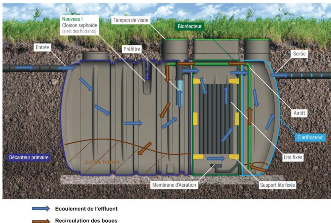
Figure 1 : Principe de fonctionnement des dispositifs STEPURBIO?
