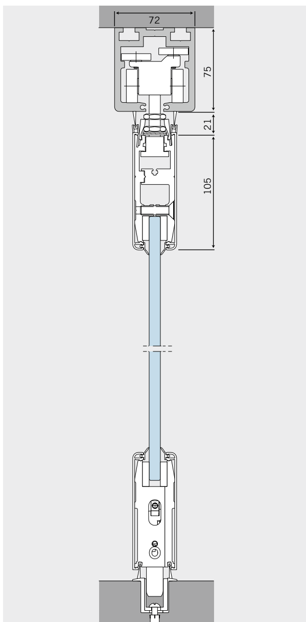
Élément de base Straightline sans profilé porteur
