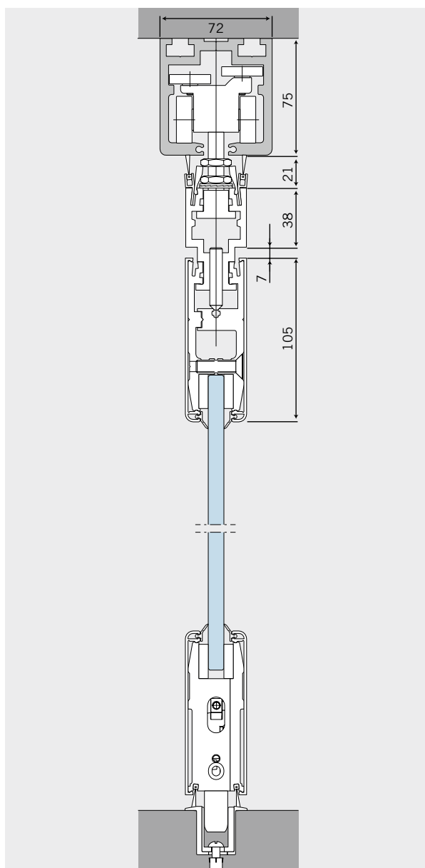
Élément de confort Straightline avec profilé porteur en cas d'exécution avec porte mobile
