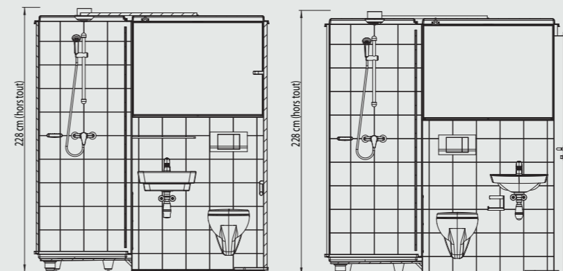
Configuration porte latérale Elevation hors tout (se référer à nos plans techniques pour détails)
