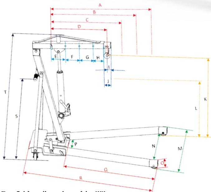
Fig. : Schéma dimensions séries WK
