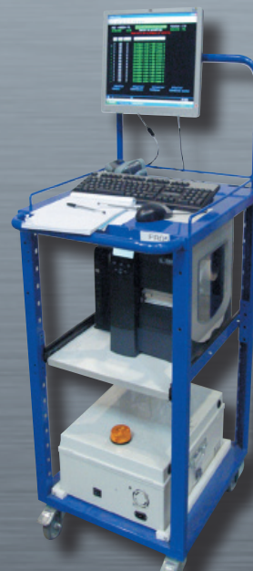
MOBIRACK avec tablette extractible avec loquet d'arrêt
