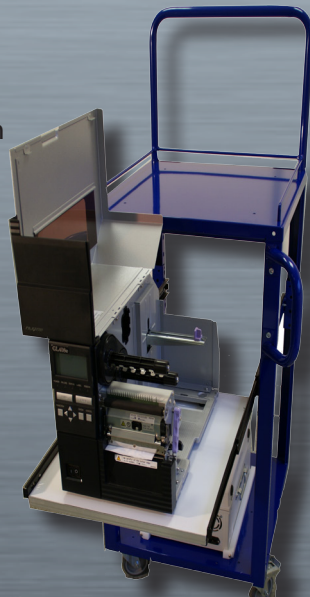
MOBIRACK avec tablette extractible avec loquet d'arrêt
