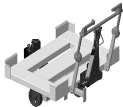
Base à assistance électrique pour fortes charges jusqu'à 2 tonnes
