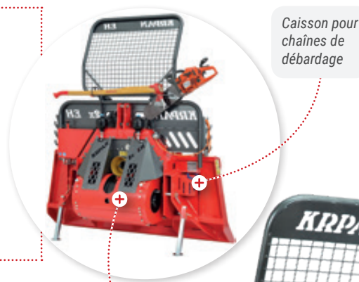
Tambour dans le sens du treuilage avec PDF centrale
