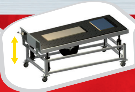
>> Table élévatrice Table à coussin d'air pour manipulation aisée des pièces lors du chargement
