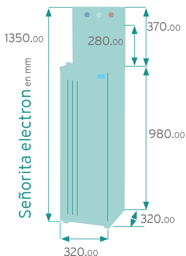
3 boutons électriques pour la distribution d'eau 3 electric buttons for water distribution
