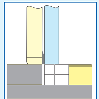
avec décaissé
