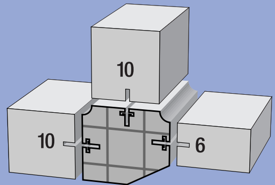
3 voies
