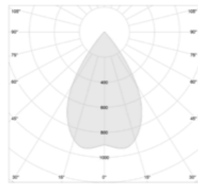
Reflector RG30 :
