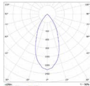
Reflector RG20 :
