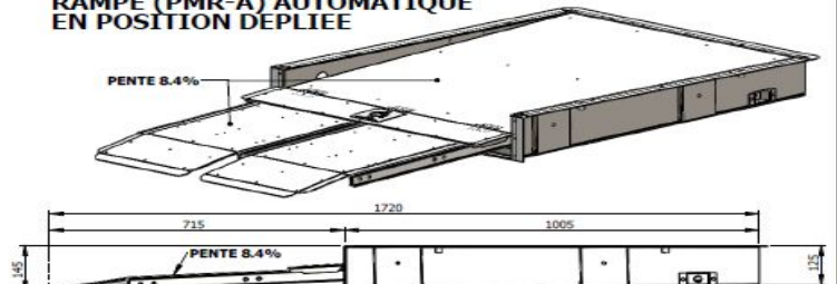
RAMPE (PMR-A) AUTOMATIQUE EN POSITION DEPLIEE
