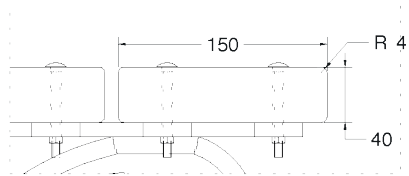
▲ Détail lames
