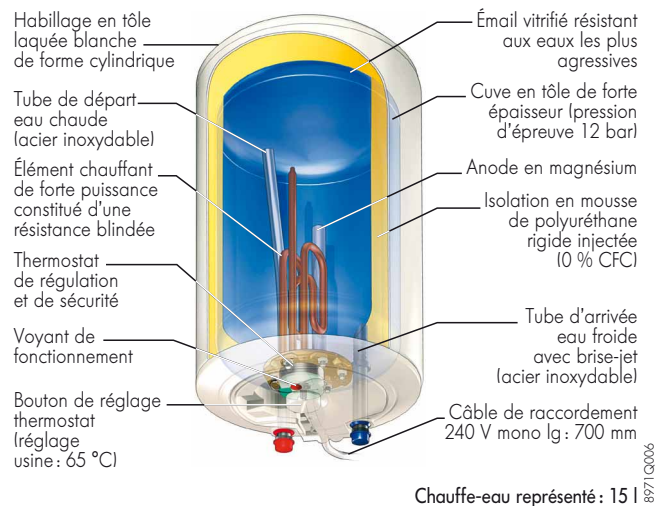
Chauffe-eau représenté : 15 l
