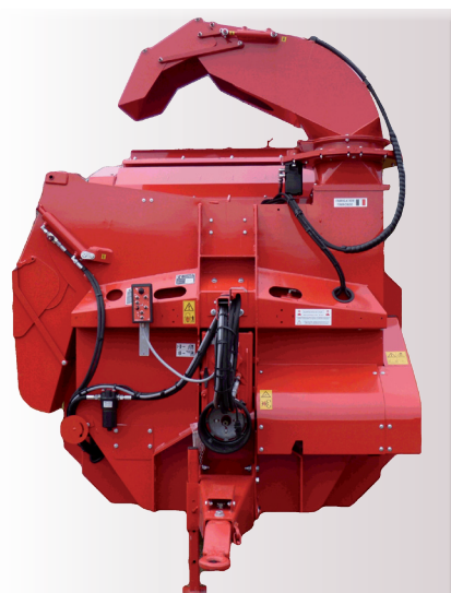
Face-avant double goulotte (conseillée pour la distribution du foin et de l'enrubannage)
