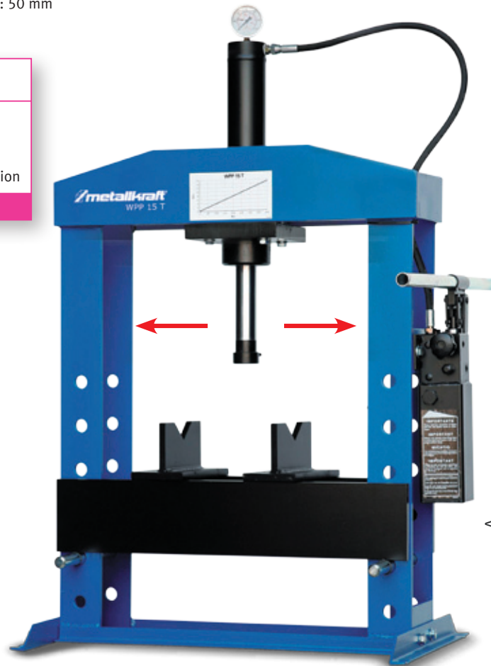
Fig.: WPP 15 T avec piston mobile
