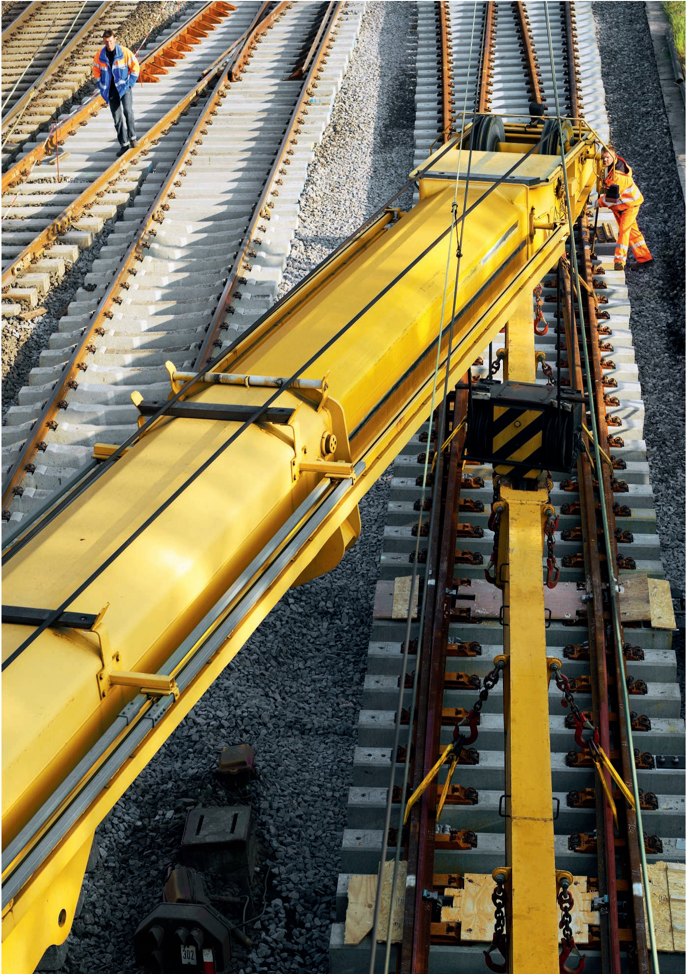
↑ Des sangles spéciales préservent les rails
