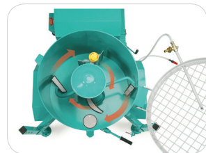
PALES DE MALAXAGE AVEC SATELLITE TOURNANT Il faut 35 secondes au MIX 360 moteur électrique pour malaxer 200 litres **.
