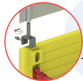
Etrier de bridage réglable facile à fixer
