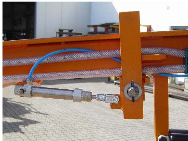
Clapet de sécurité automatique
