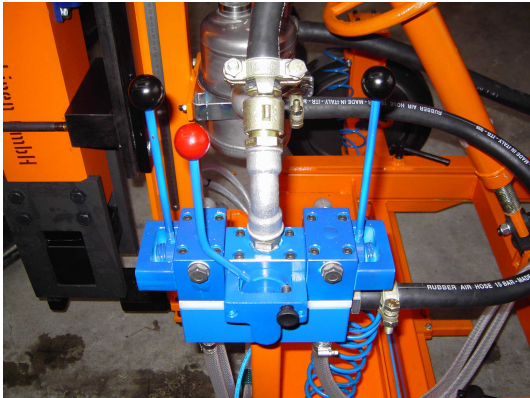
Bloque de commande pour opérer le palan, marteau batteur, entraînement et frein à air comprimé
