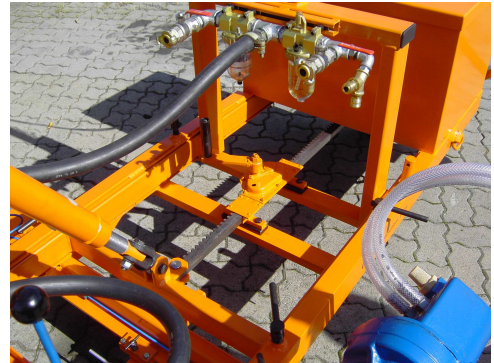
Séparateur d'eau avec huileur pour consommateur p. ex. tournevis à frapper, treuil d'avancement et vis à garrot
